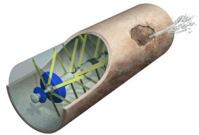
그림12 뉴보텍 비굴착보수공법(OCR) 시공상황도
