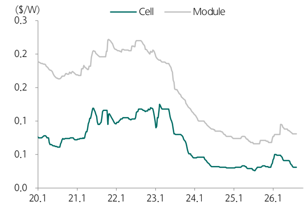
도표 17. 중국 셀/모듈 가격 추이
