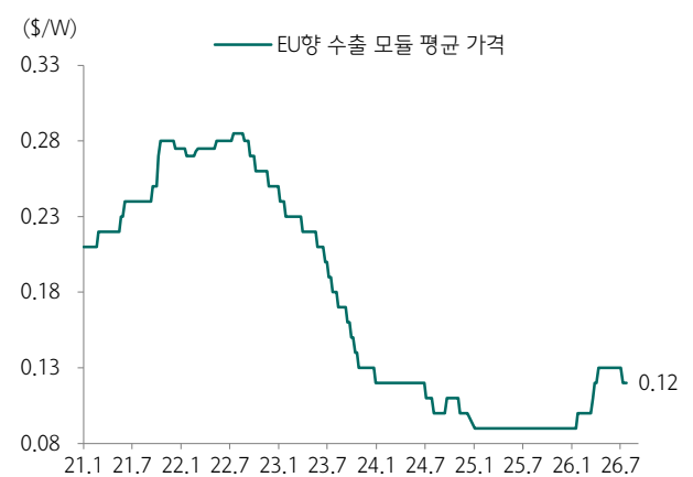
도표 28. 중국의 EU향 수출 모듈 평균가격 추이
