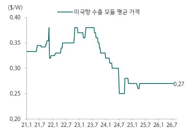
도표 29. 중국의 미국향 수출 모듈 평균가격 추이
