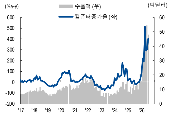
그림20. 컴퓨터 +404%
