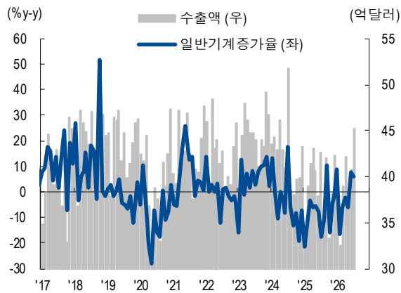
그림25. 일반기계 +6%
