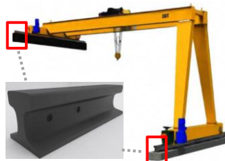
[크레인 레일]
