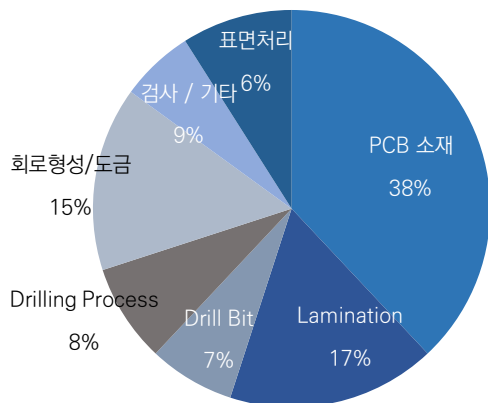
[도표 03] 고다층 PCB 제조원가 추정
