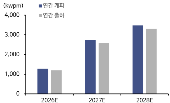
TSMC CoWoS 연간 캐파, 출하 전망
