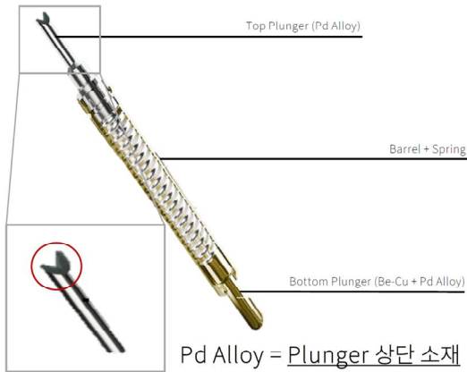
그림13. Pd Alloy 제품
