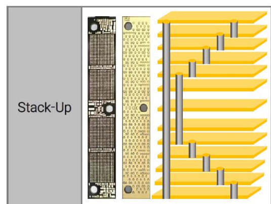
그림7. 5회 적층(SOCAMM) 공정
