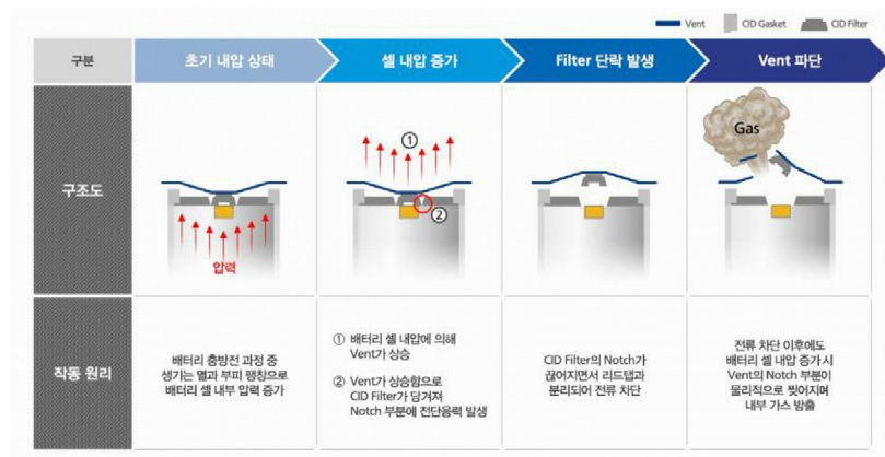
[그림 11] Topcap Ass'y 작동 원리
