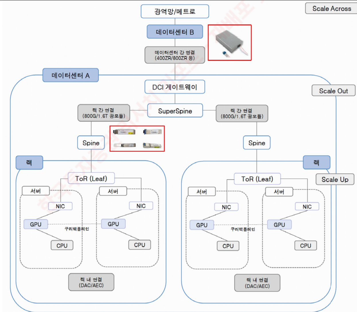
[그림 7] PnP 증폭기 수요처: 데이터센터 내 고대역폭 증폭 / DWDM 수요처: DCI/스케일업크로스 장거리 증폭 구간 적용
