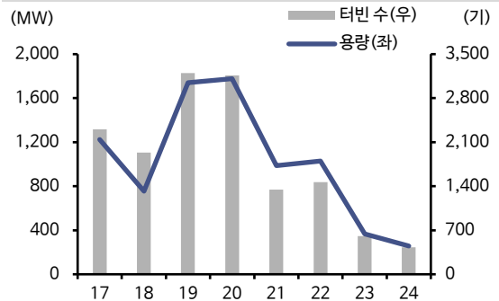
미국 부분 리파워링 추이
