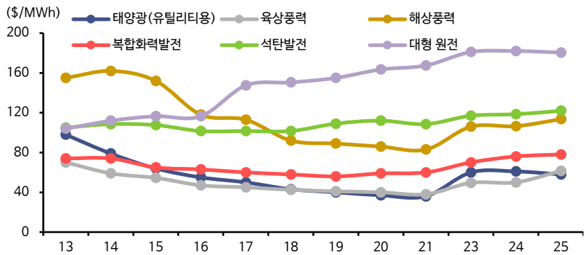
주요 발전원별 LCOE 추이
