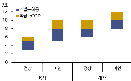
풍력 프로젝트 단계별 소요기간
