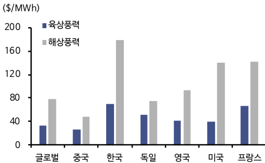
주요국 풍력발전 LCOE 비교
