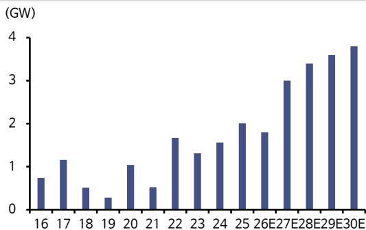
유럽 리파워링 용량 추이 및 전망
