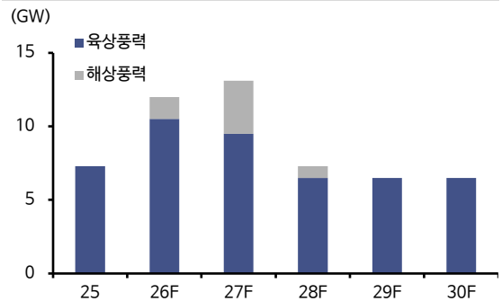
북미 풍력 신규 설치 전망
