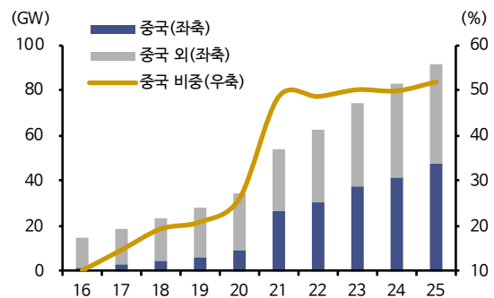
글로벌 해상 풍력 누적 설비 추이
