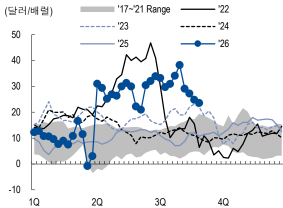
그림9. 휘발유 정제마진
