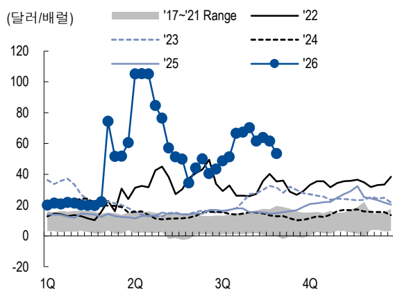
그림11. 항공유 정제마진
