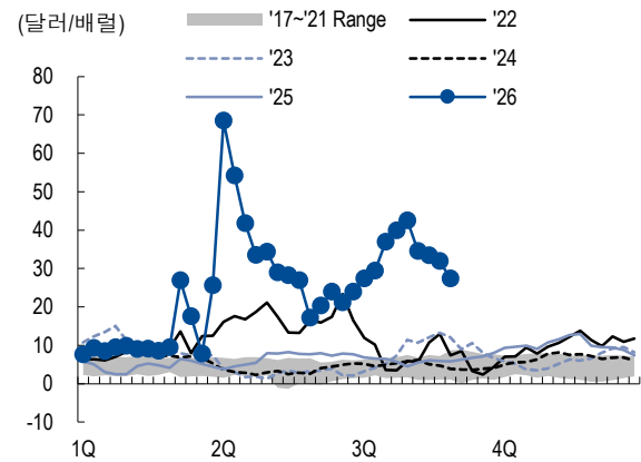
그림8. 국내복합정제마진
