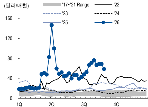
그림10. 경유 정제마진
