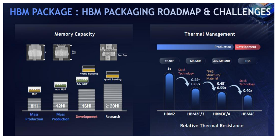
그림 4. SK하이닉스 HBM 패키징 로드맵
