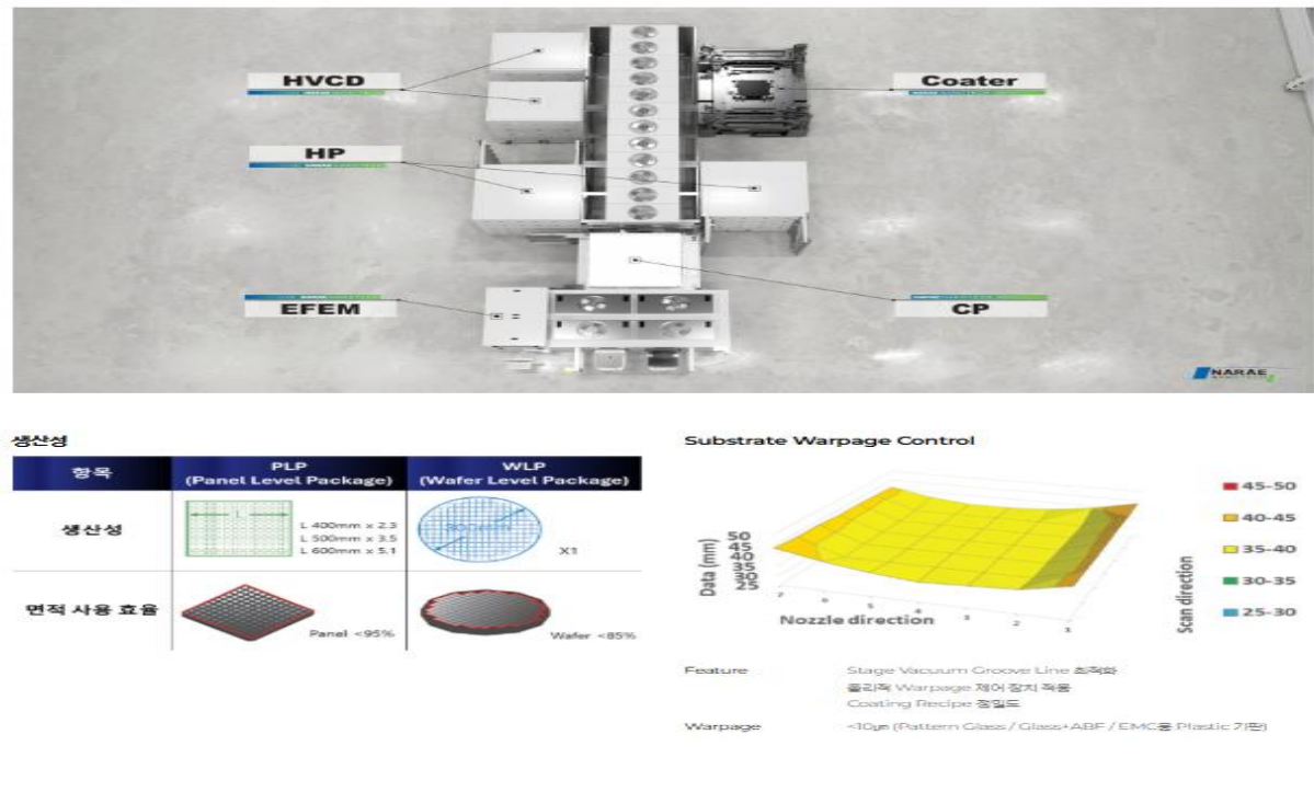
그림 3. PLP-Panel Level Packaging Line
