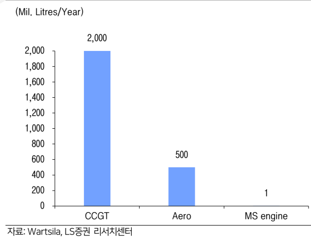
그림27 300MW Off-grid DC 냉각수 소비량
