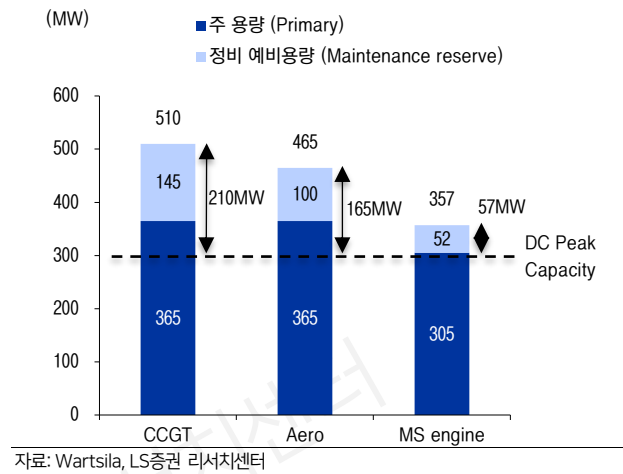
그림25 300MW Off-grid DC 설비 필요용량
