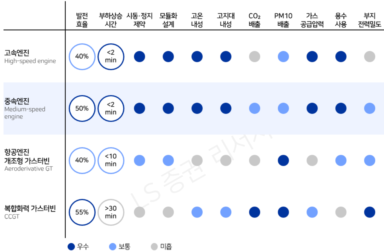
그림20 DC 주전원용 주요 On-site 설비 비교(Wartsila)
