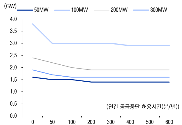
그림19 1GW DC 전원용 가스터빈 설비용량(가동률 85%)
