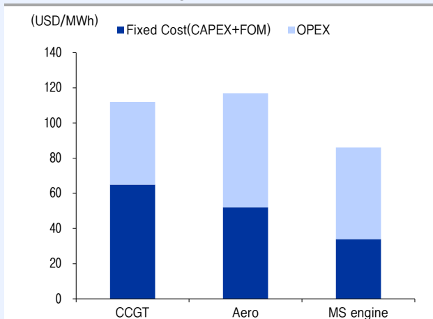
발전원별 300MW Off-grid DC 발전단가 비교
