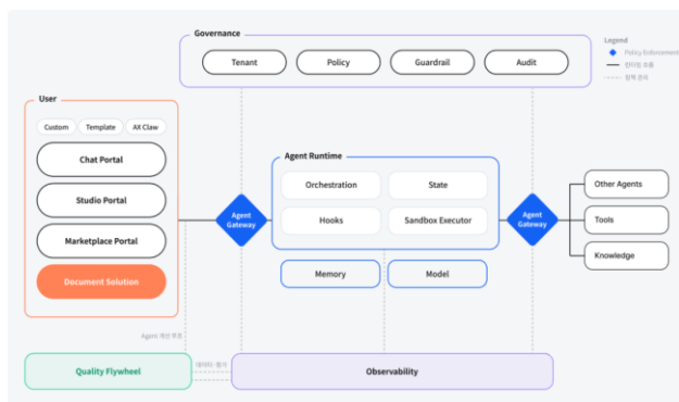
그림 5 _ 소버린 에이전틱 OS 구조
