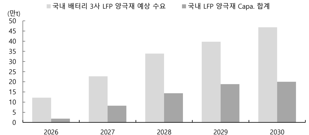
국내 배터리 3사 LFP 양극재 예상 수요와 국내 LFP 양극재 캐파 비교
