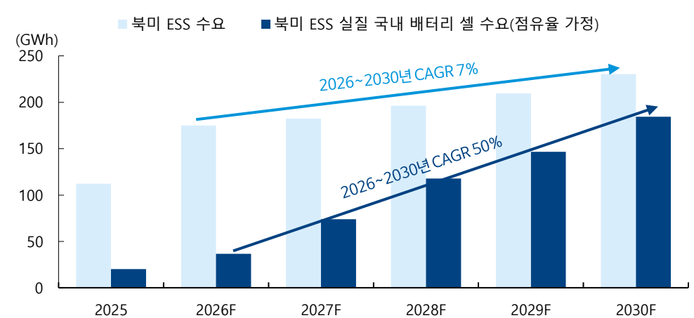
북미 ESS 수요와 PFE 규제로 인한 점유율 가정 반영한 한국 ESS 배터리 실질 수요 전망
