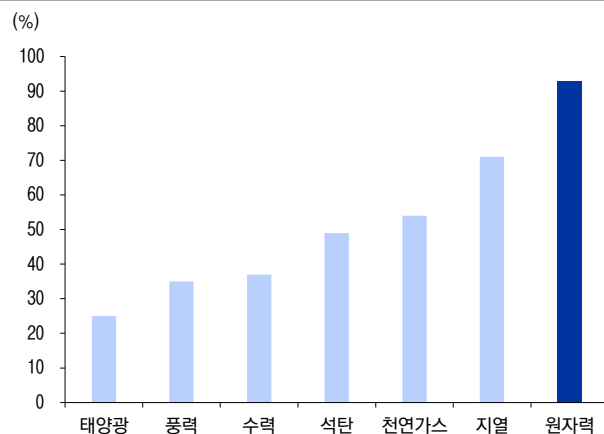
그림30 발전원별 가동률
