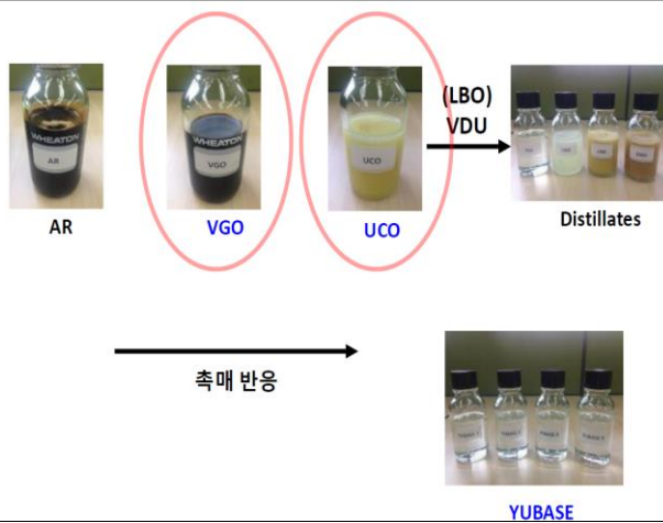
그림 11 윤활기유 제조 공정: 원료, 중간재, 제품
