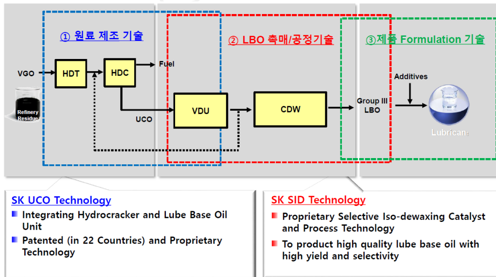
그림 14 SK 윤활기유 제조 공정 및 핵심기술(UCO 및 SID 기술)
