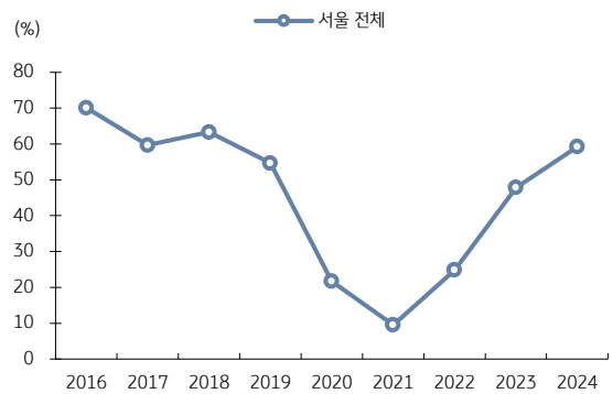
그림 11. 서울 전체 외국인 숙박객 비율
