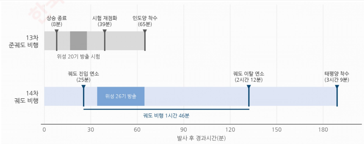
[그림 4] 13차와 14차 비행 타임라인 비교
