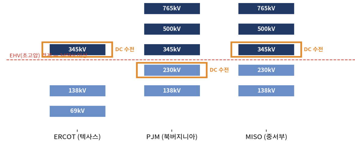
그림 11. 미국 주요 계통운영기관의 송전 전압 체계와 고압(HV)/초고압(EHV) 송전망
