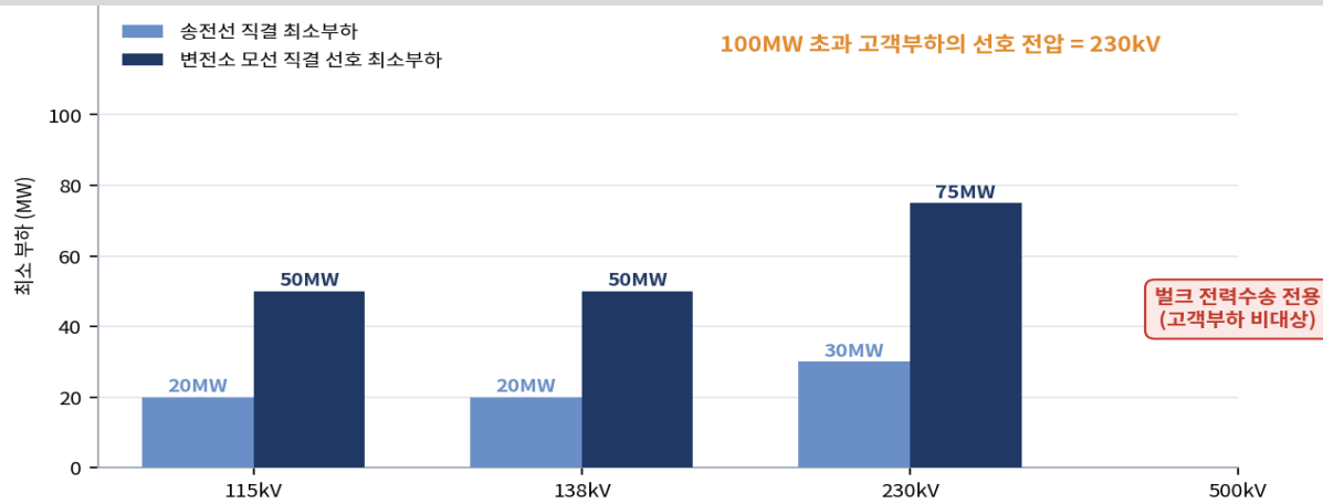
그림 10. 미국 Dominion Energy Virginia 의 전압별 대형부하 직접 접속 기준
