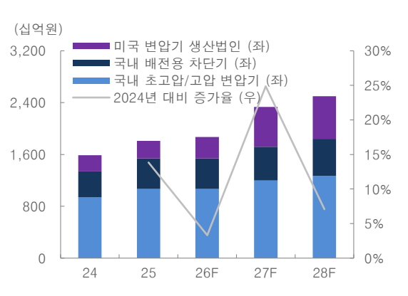
그림 6. HD 현대일렉트릭의 변압기 생산능력 전망
