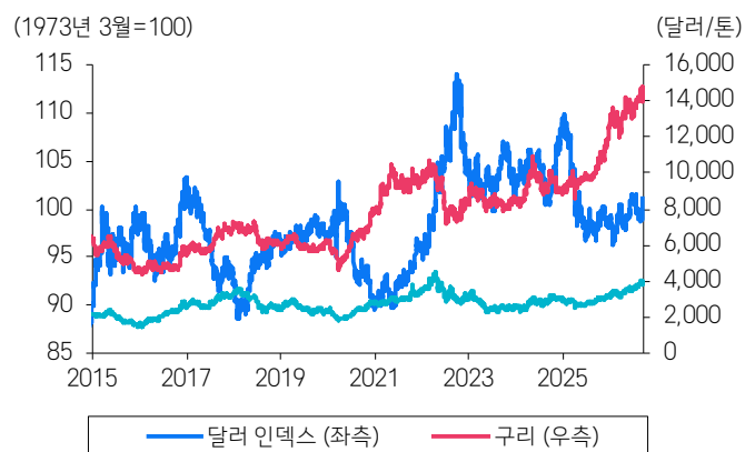
달러 인덱스 vs 구리 및 아연 가격
