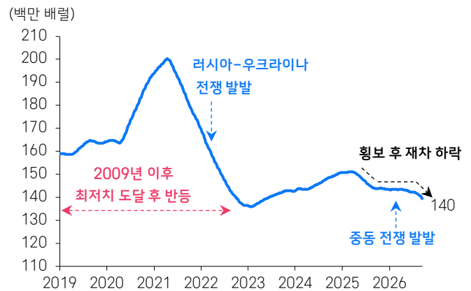
글로벌* 등경유 재고** 추이
