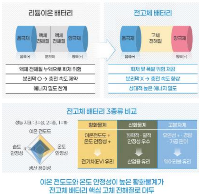
그림 1 전고체 배터리
