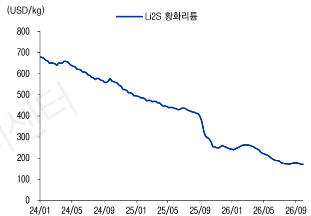
그림 7 황화리튬(황화물계 전해질 원가 80~90%) 가격 추이
