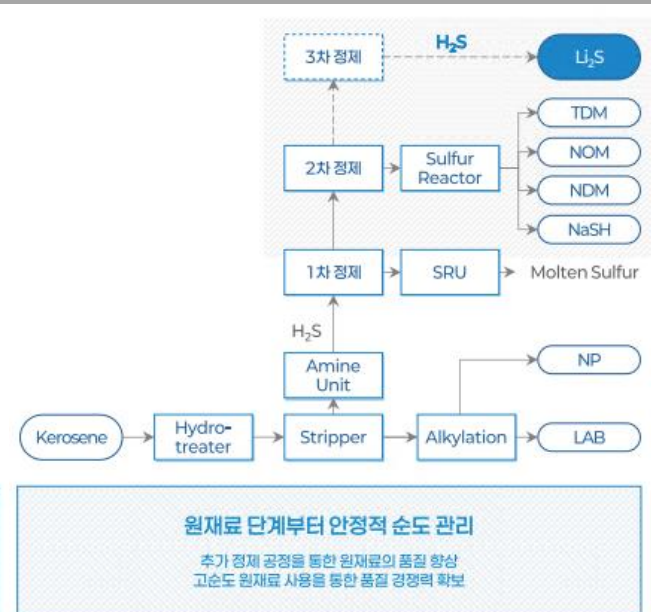
그림 4 동사 경쟁력 중 하나인 황화수소 순도 관리
