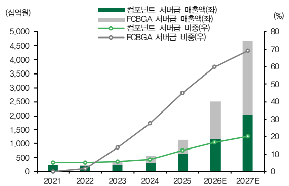
도표 18. 삼성전기 서버함 매출 추이, 비중 추이
