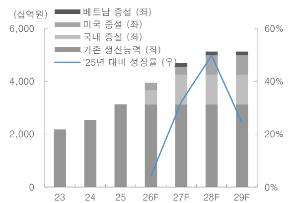
그림 2. 효성중공업 변압기 생산능력 전망
