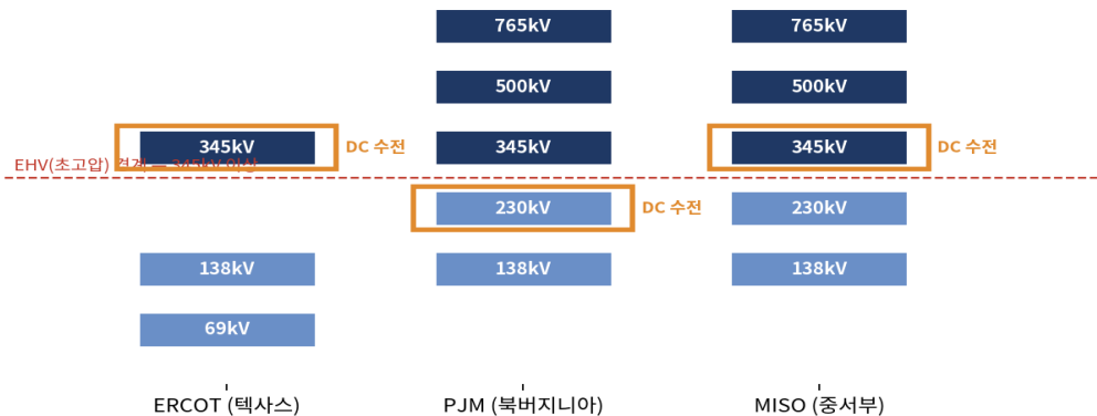
그림 11. 미국 주요 계통운영기관의 송전 전압 체계와 초고압(EHV) 구간
