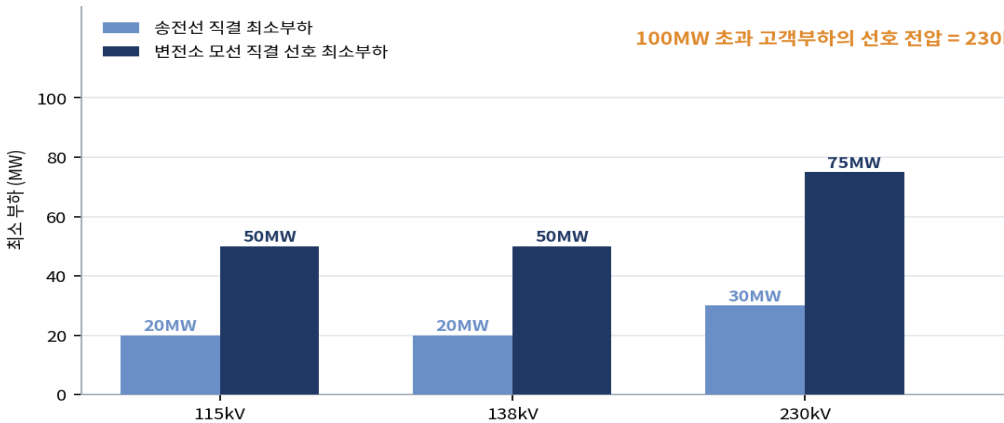
그림 10. 미국 Dominion Energy Virginia 의 전압별 대형부하 직접 접속 기준
