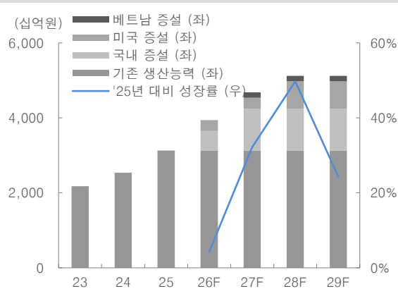
그림 2. 효성중공업 변압기 생산능력 전망
