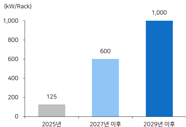
그림5 800VDC 이후 서버랙당 전력 부하 지속 상승
