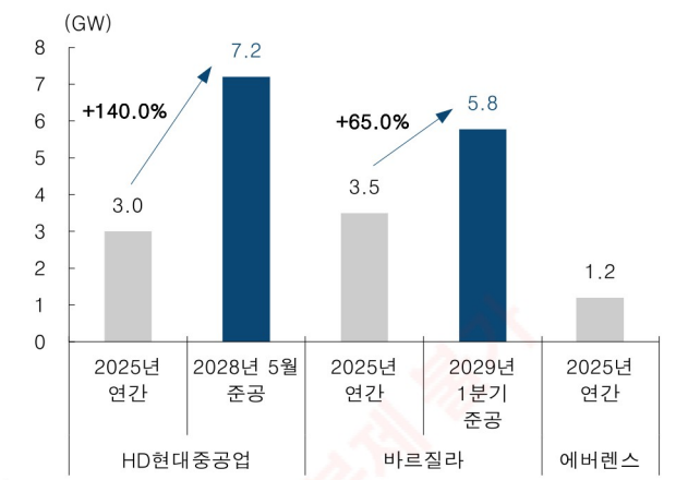
[그림 2] 4행정 중속엔진 Licensor 3사 생산 시설 용량
