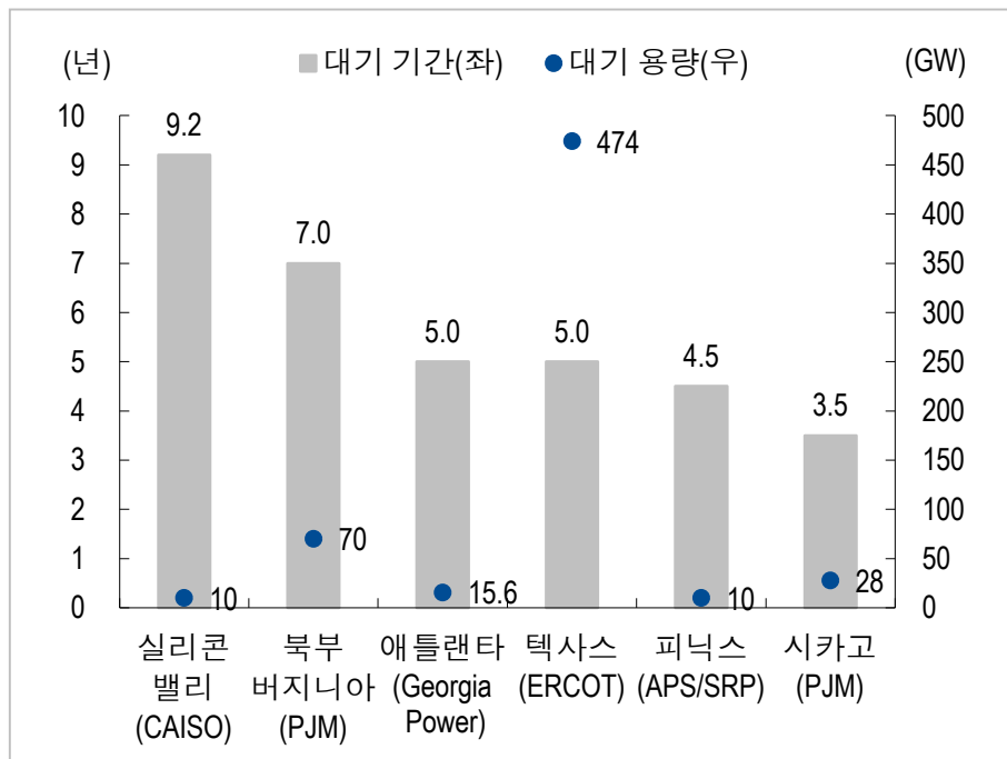
북미 주요 데이터센터 허브별 전력 계통 대기 기간 및 용량
