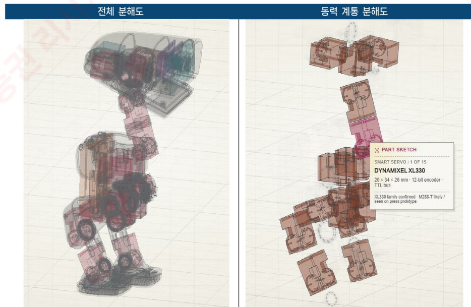
&lt;표 2&gt; 마이크로덕 분해도: 로봇티즈 다이내믹셀 XL330
