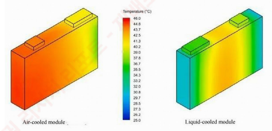
[그림 6] 액체냉각 기반 BESS와 공랭식 BESS 비교
