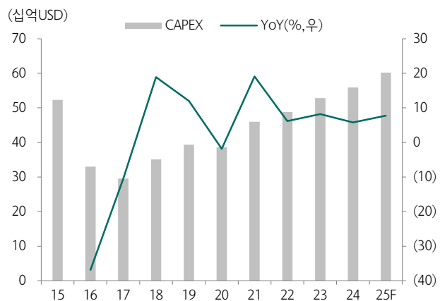
도표 38. 글로벌 주요 광산기업들의 CAPEX 추이
