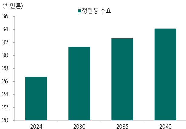
도표 37. 중장기 정련동 수요 전망
