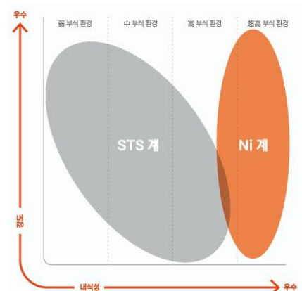
그림25. 니켈합금의 높은 내식성
