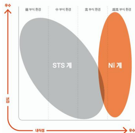
그림63. 니켈합금의 높은 내식성(부식저항성)
