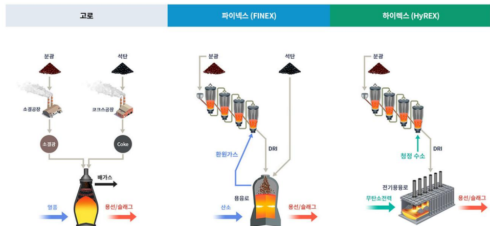
그림16. POSCO홀딩스는 저탄소 철강 기술(석탄 대신 수소를 환원제로 사용하는 기술) 개발 중
