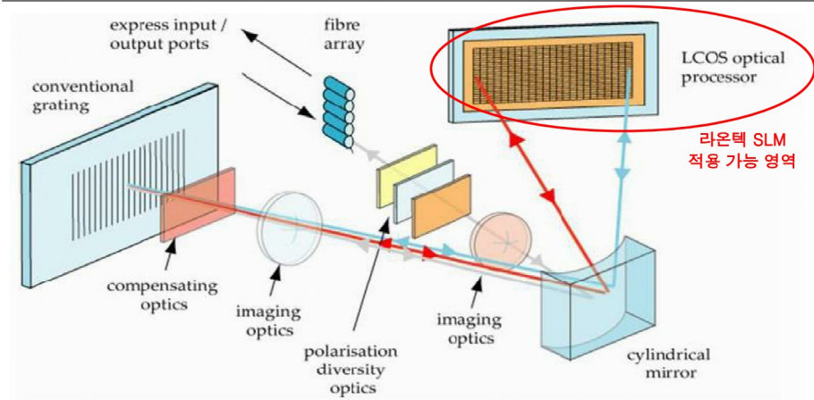
[그림 11] LCoS 기반 WSS 도식: 파장별 광경로를 제어해 원하는 출력 포트에 스위칭
