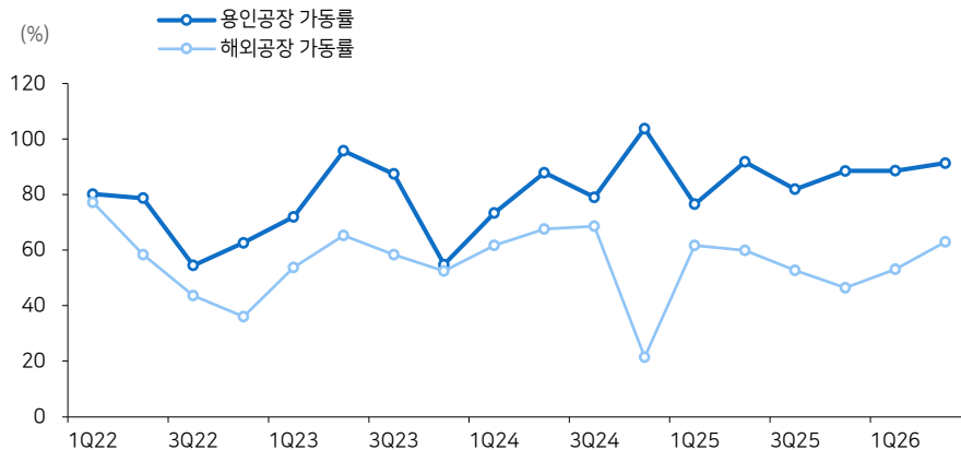
그림4 삼화콘덴서 국내/해외 공장 가동률 추이
