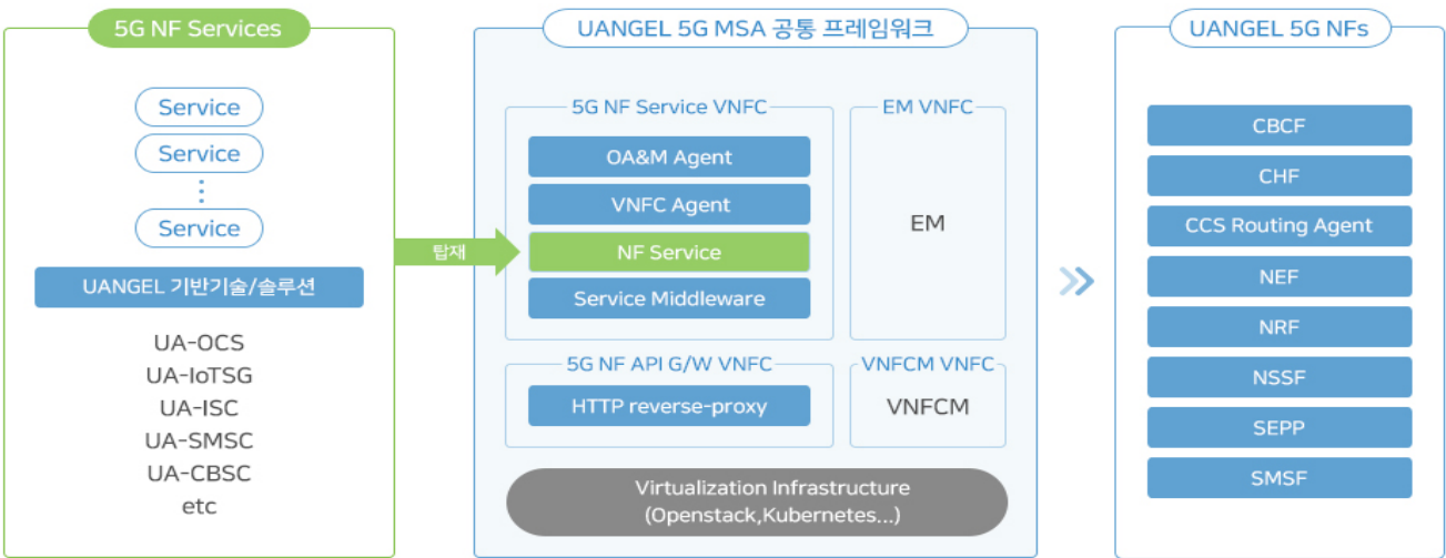
그림3 유엔젤 5G 기반 코어네트워크
