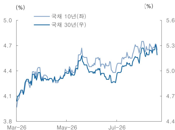
[그림 6] 美 장기 금리 단기적 고점, 하락은 기대인플레이션 연동
