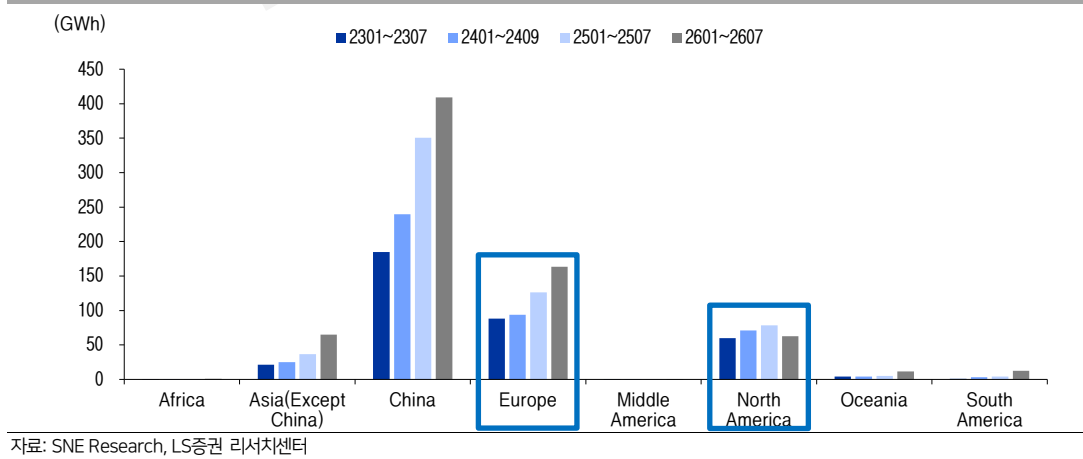
그림 4 글로벌 EV 배터리 추이(1~7월, 지역별)
