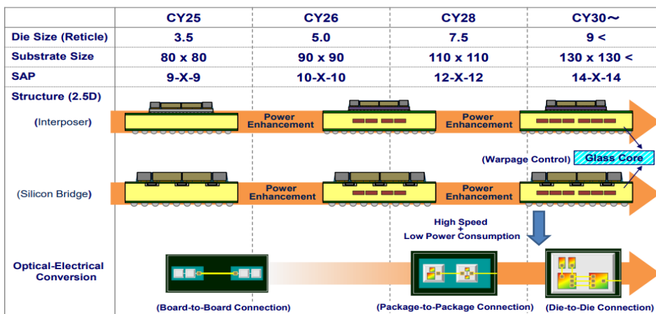
그림7 ABF 기판 기술 로드맵
