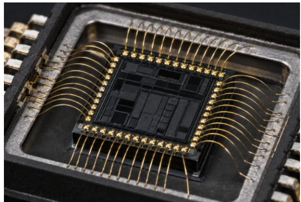
[도표 04] 골드 본딩 와이어
