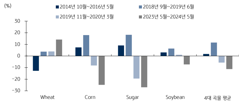
그림 31. 오히려 최근 2회 엘니뇨 동안 밀을 제외한 곡물 가격 하락
