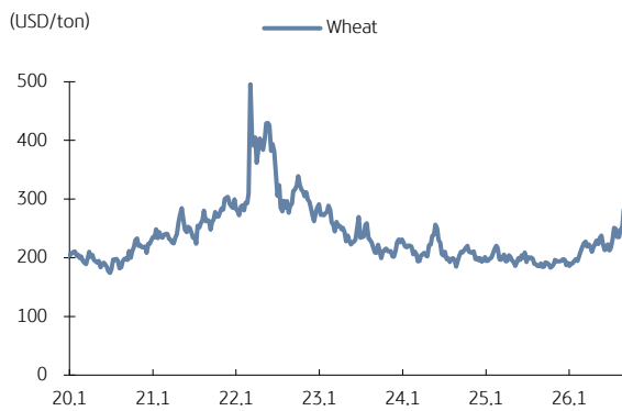
그림 26. 밀 가격 톤당 280달러로 상승했으나 2023년 수준
