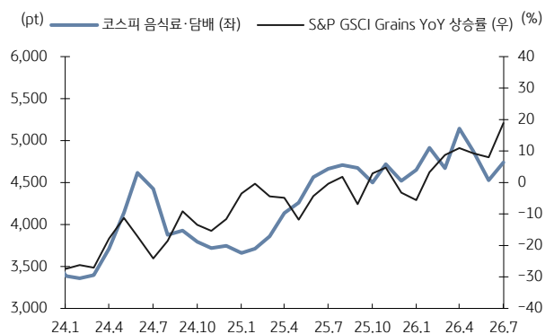
그림 13. 코스피 음식료·담배 지수와 곡물 가격 상승률은 동행
