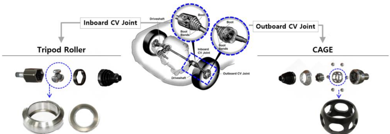
도표 15. Cage, tripod roller 구동원리
