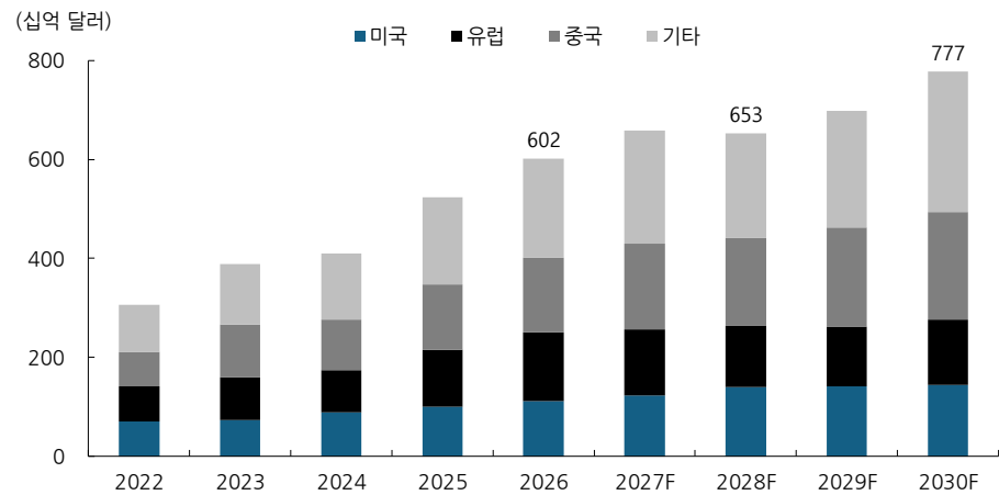
그림3 글로벌 전력망 투자액 전망
