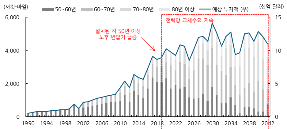
그림4 예상 교체 규모 감안 시 대규모 투자 필요
