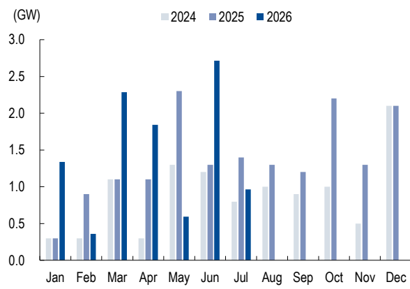
그림4. 미국 ESS 월별 설치 용량
