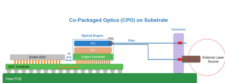
[그림 4] ELSFP(External Laser Source Formpacter)는 CPO 내 외부광원 역할
