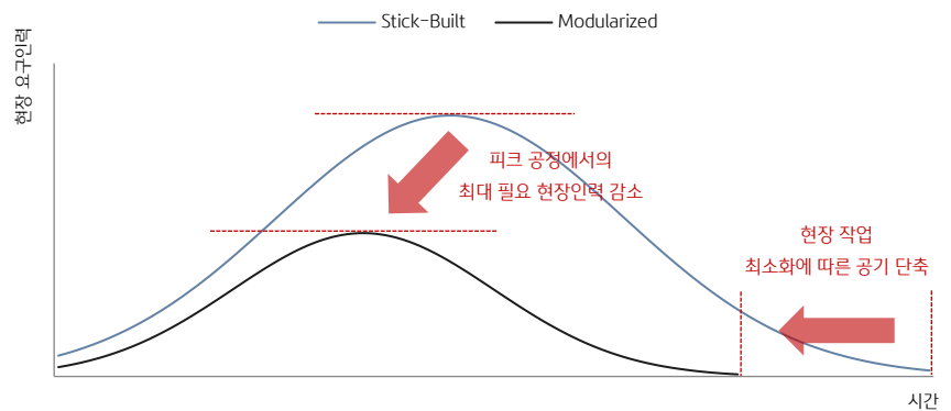
그림 36. Stick-Built 방식과 모듈러 방식의 공기 및 현장 요구인력 비교
