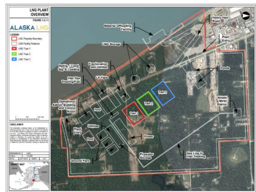
그림 34. 알래스카 LNG 프로젝트 플랜트 배치도
