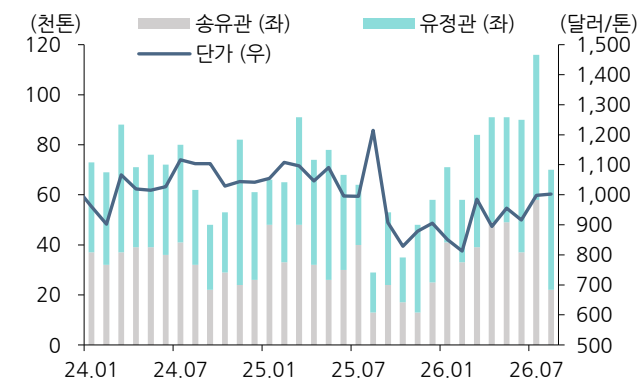
그림 5. 국내 월별 유정관 및 송유관 수출물량
