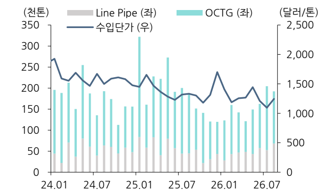
그림 6. 미국 월별 유정관 및 송유관 수입물량
